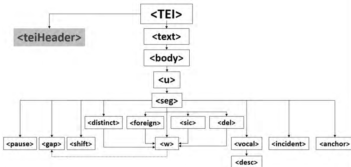
Figura 4: struktura XML fajla vezana za hijerarhijsku organizaciju i anotaciju teksta
