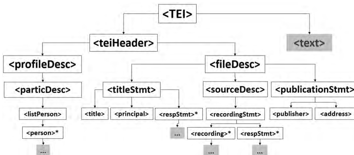
Figura 3: Osnovna struktura zaglavlja TEI XML fajla u ITALSERB korpusu
