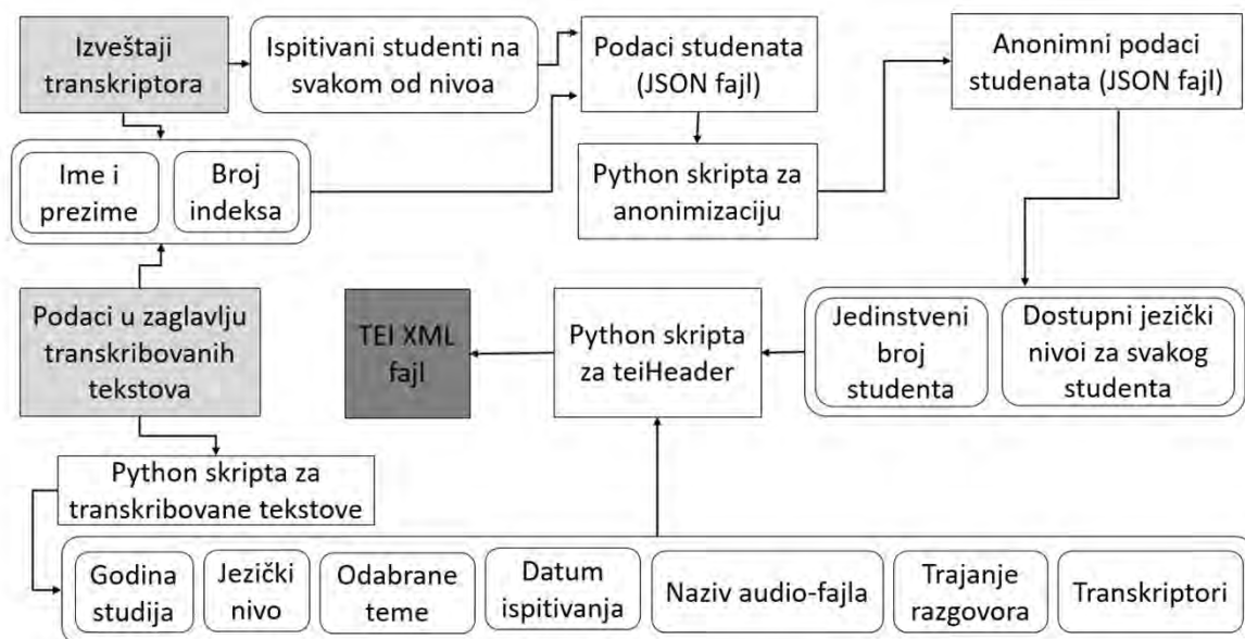
Figura 2: Vizuelni prikaz procesa obrade metapodataka u ITALSERB korpusu
