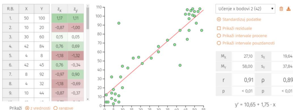
Slika 47. Dijagram raspršenja koji prikazuje visoku povezanost dužine učenja u satima i broja bodova osvojenih na testu znanja
