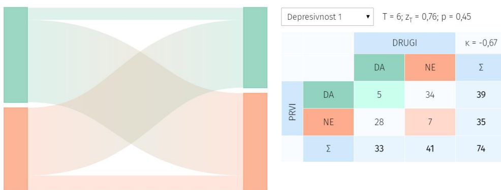
Slika 58. Primer u kome Maknimarov test sugerise da nema razlike između dva merenja dok Koenova kapa pokazuje da ne postoji saglasnost
